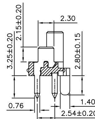
① Section A-A
